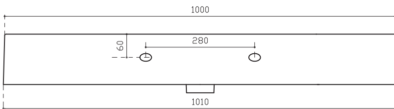
Vista dall'alto Top View
